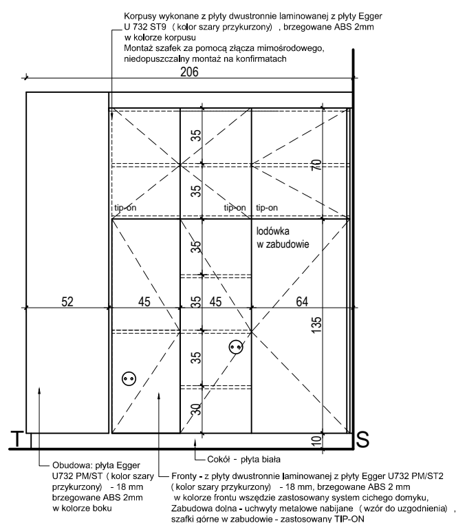
KUCHNIA 1.11 widok T-S
