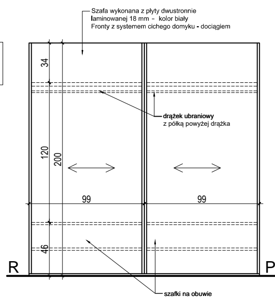
SZATNIA 1.12 widok R-P
